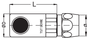
Coupling for Rubber Tube Kupplung für Kunststoffschlauch
