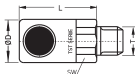
Coupling Male Thread Kupplung mit Aussengewinde
