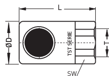
Coupling Female Thread Kupplung mit Innengewinde
