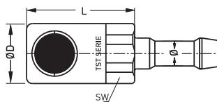
Coupling for Rubber Hoses Kupplung mit Schlauchanschluss
