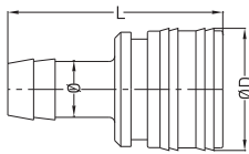
Hose Tail Coupling Without Valve Kupplung mit Schlauchtülle ohne Ventil
