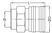
Female Thread Coupling Without Valve Kupplung mit Innengewinde ohne Ventil
