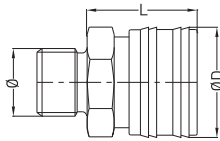
Male Thread Coupling Without Valve Kupplung mit Aussengewinde ohne Ventil
